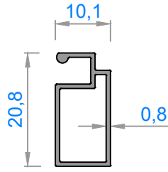
1727 - 0,143 kg/m
