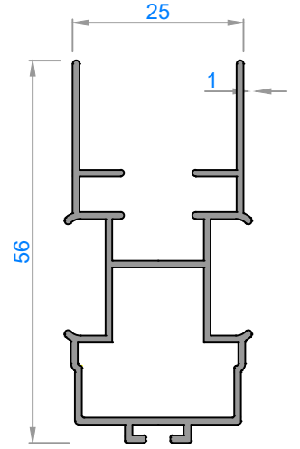
4474 - 0,395 kg/m
