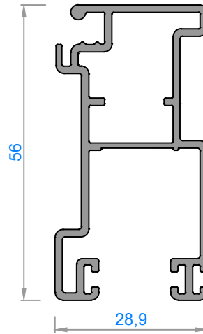
4731 - 0,800 kg/m
